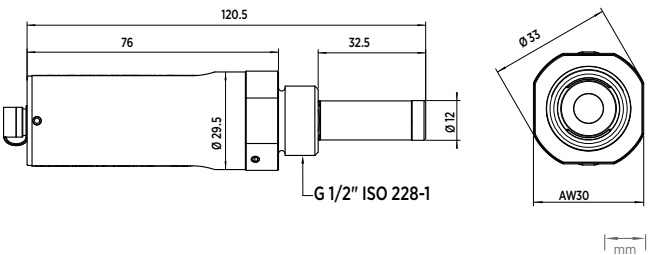
DMT152 尺寸
