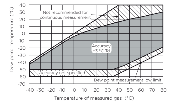
DPT145 露点测量准确度
