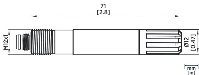
HMP110 探头
