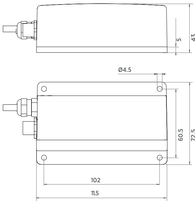
HMT310 变送器本体
